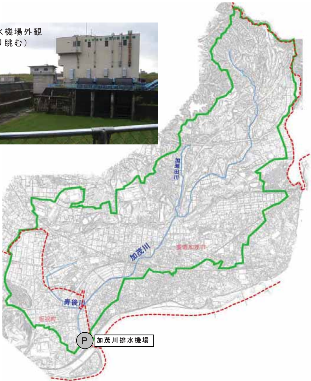
図- 2.1.8 加茂川排水機場位置図
