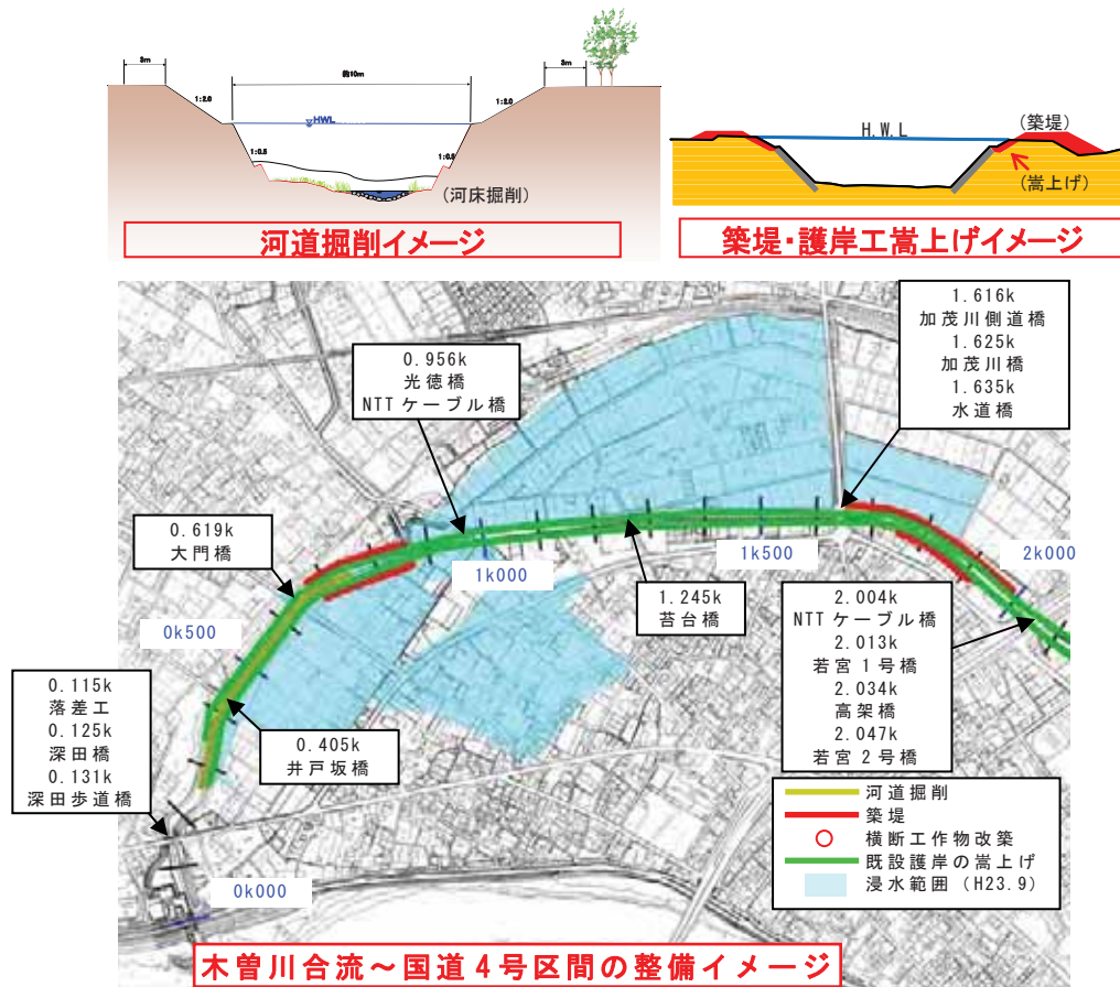
図- 3.6.21 加茂川改修イメージ
