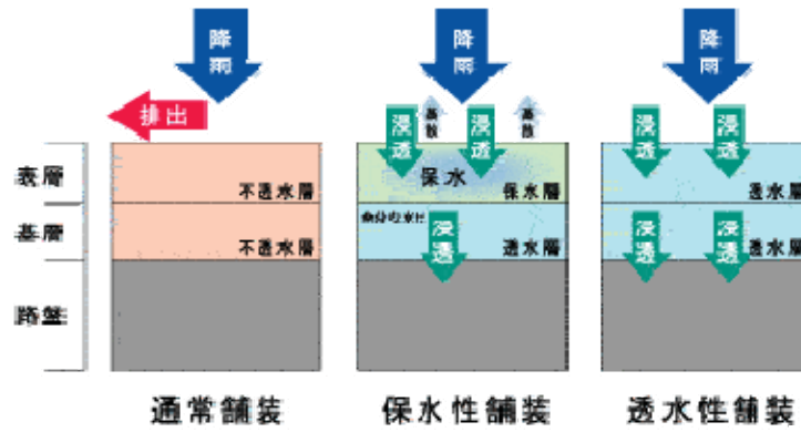
図- 3.6.18 雨水貯留浸透施設のイメージ
