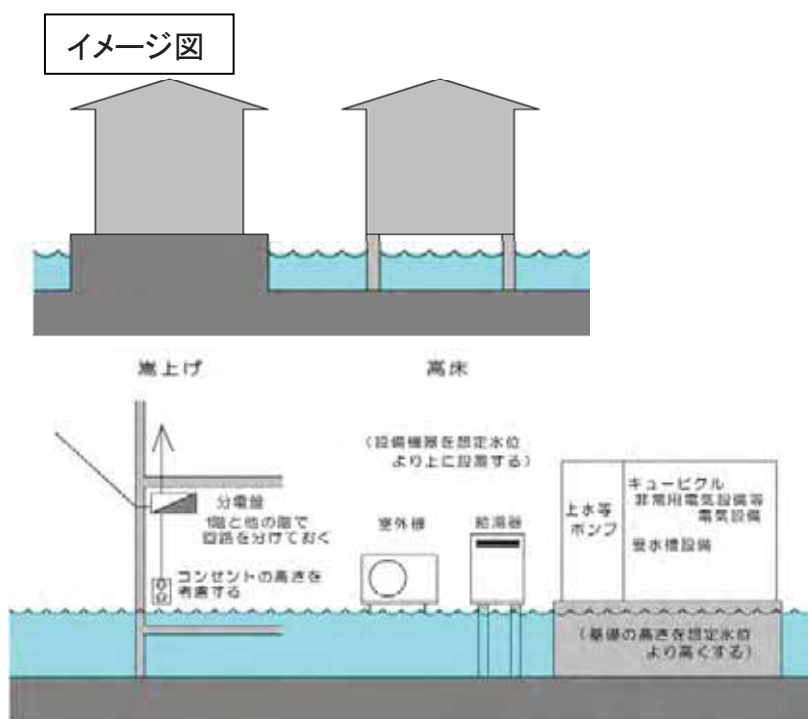
図- 3.6.9 建築高さ等のイメージ
