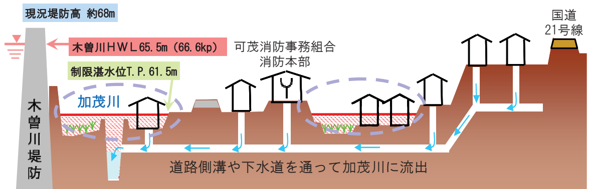
図- 2.1.4 対象区域の地形的特徴（断面横断模式図）
