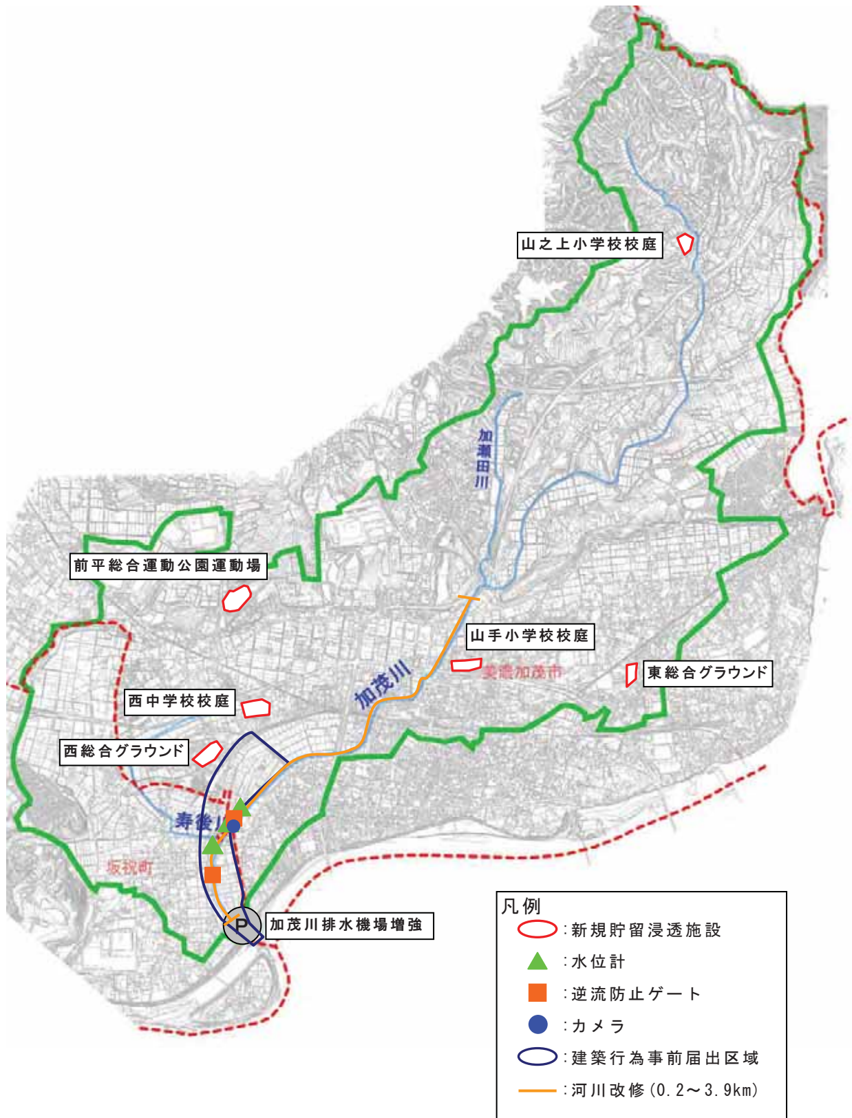
図- 3.6.24 内水対策計画実施位置図
